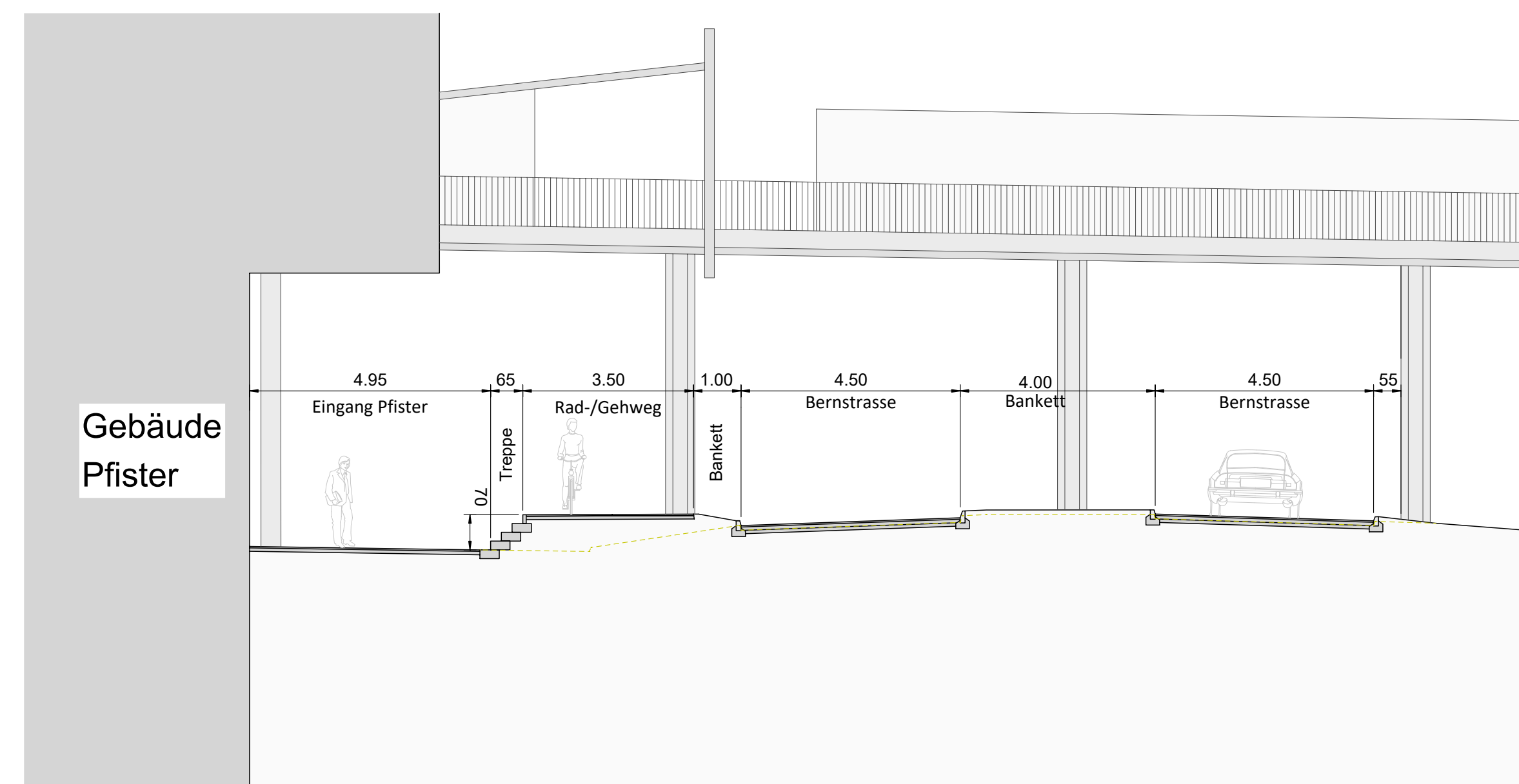
Schnitt 2 - 2 1:100
