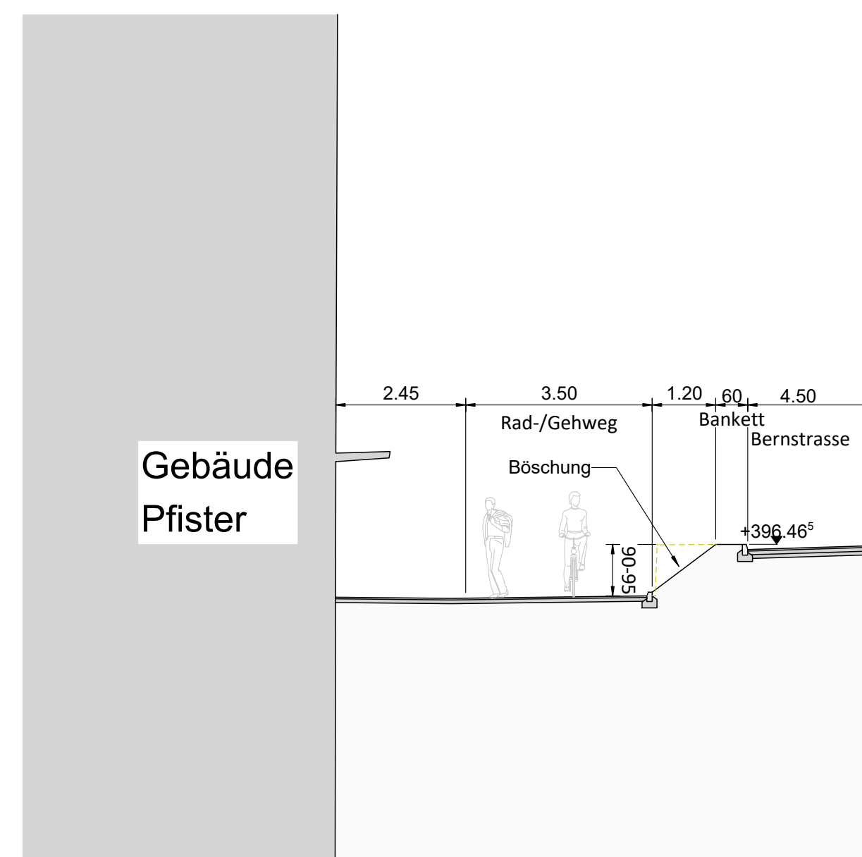
Schnitt 1 - 1 1:100
