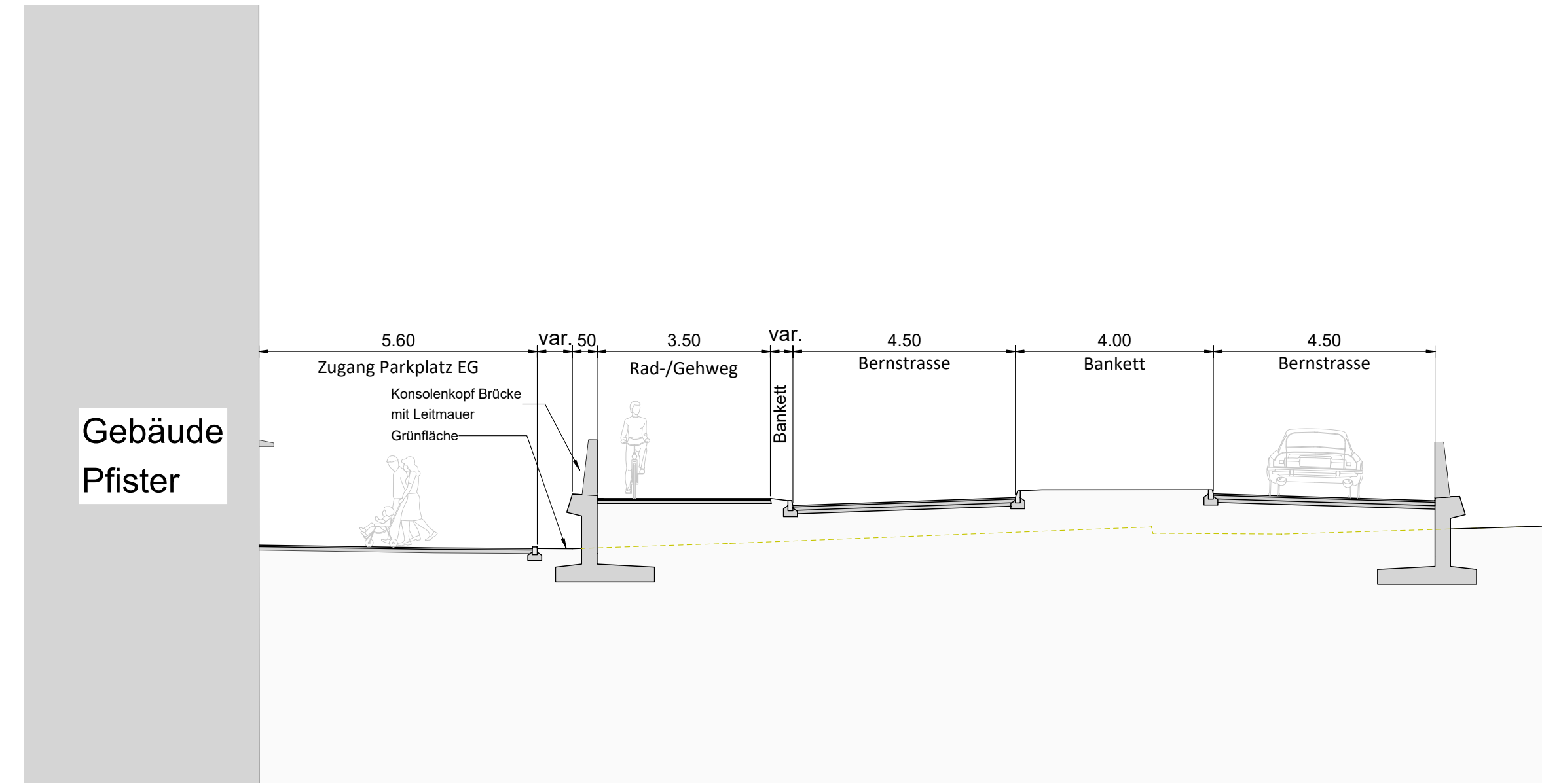
Schnitt 3 - 3 1:100
